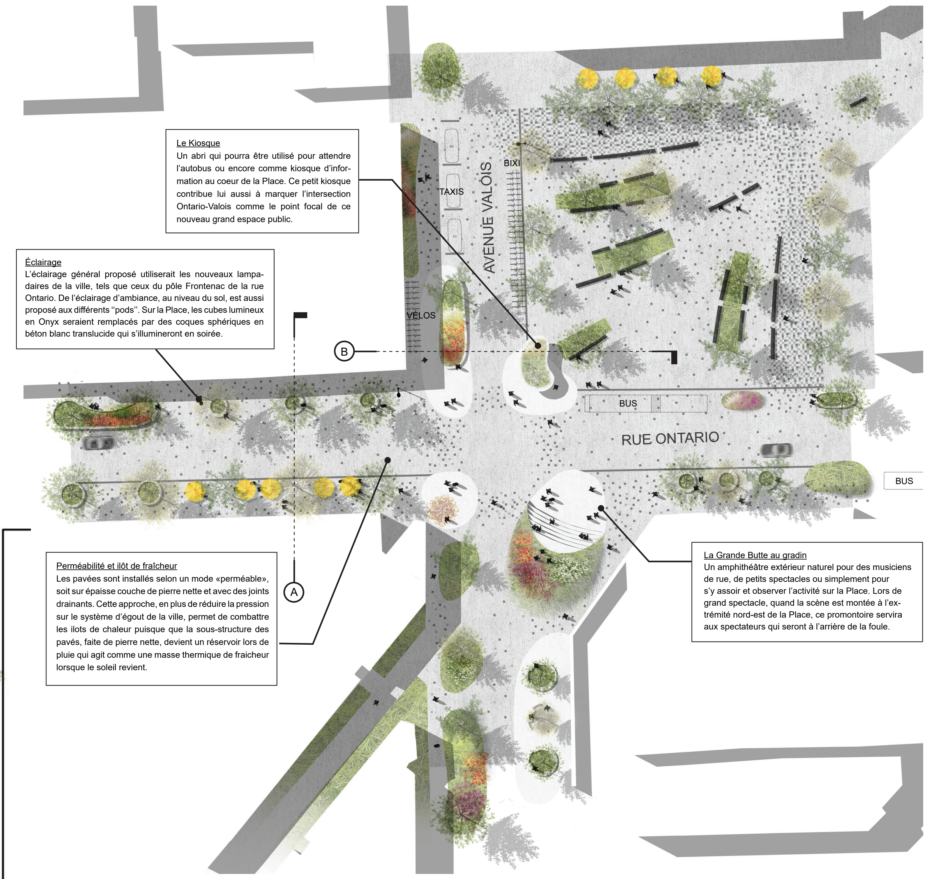
PLAN DE L'INTERVENTION PROPOSÉE 1:300
