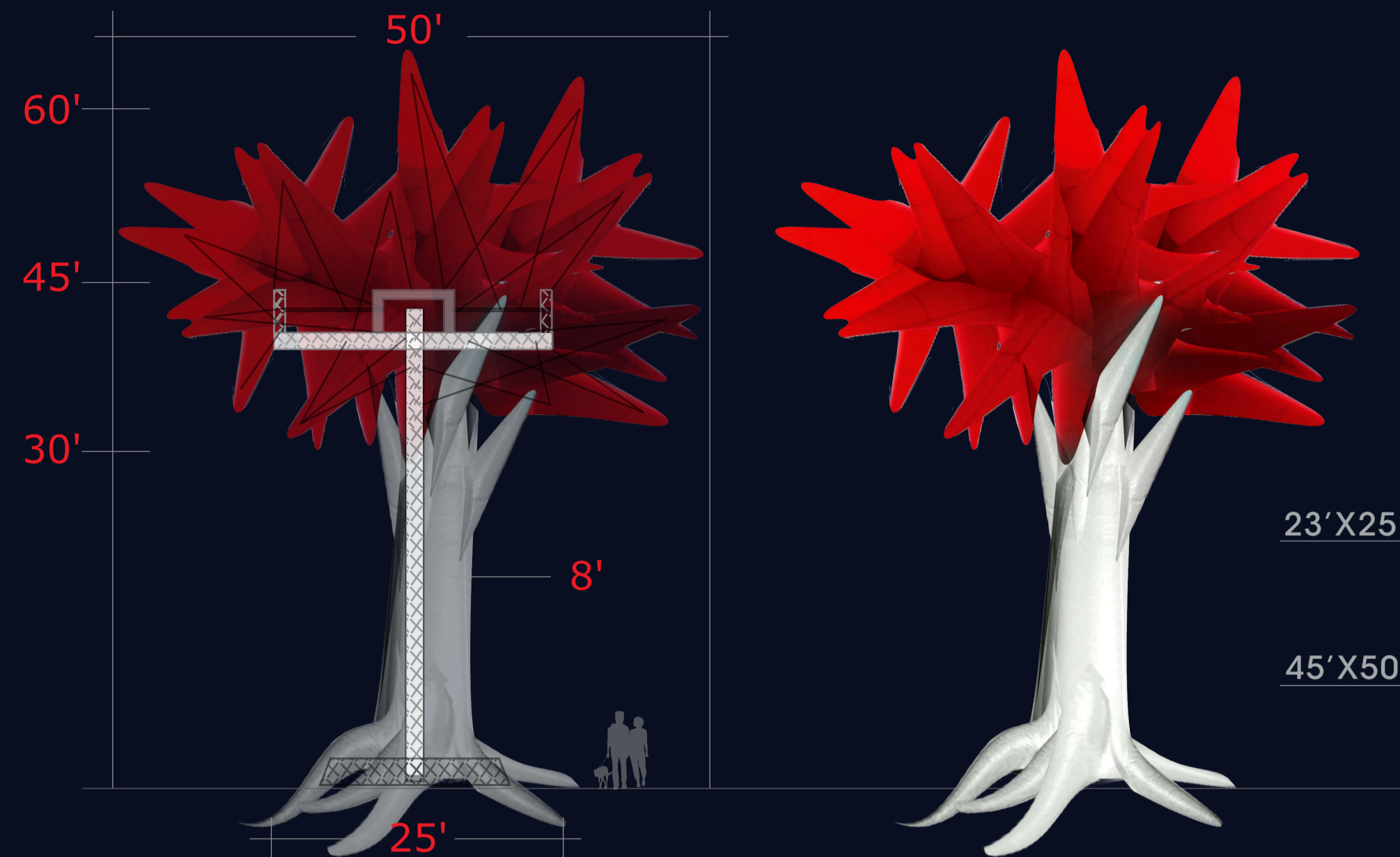
La structure permet l'installation d'une nacelle pouvant accueillir adéquatement les systèmes techniques et l'encrage du "feuillage".
