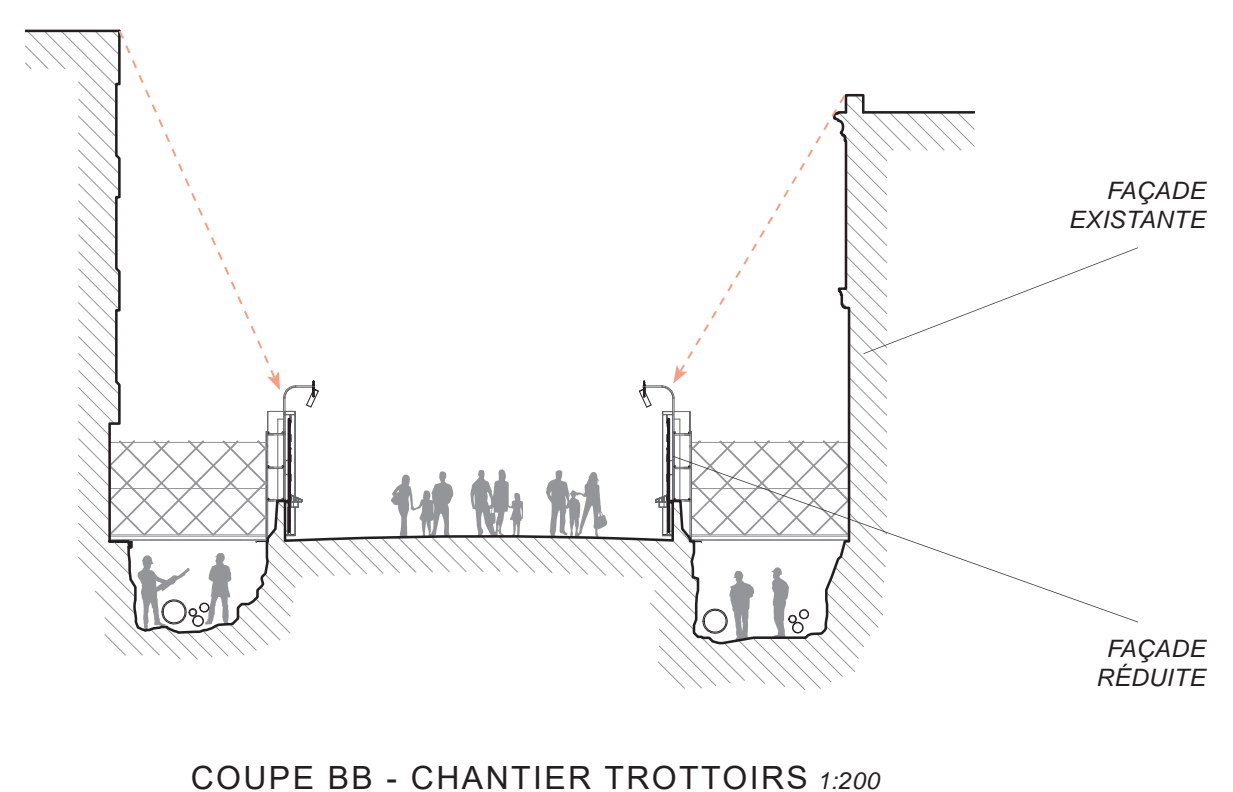
COUPE BB - CHANTIER TROTTOIRS 1:200
