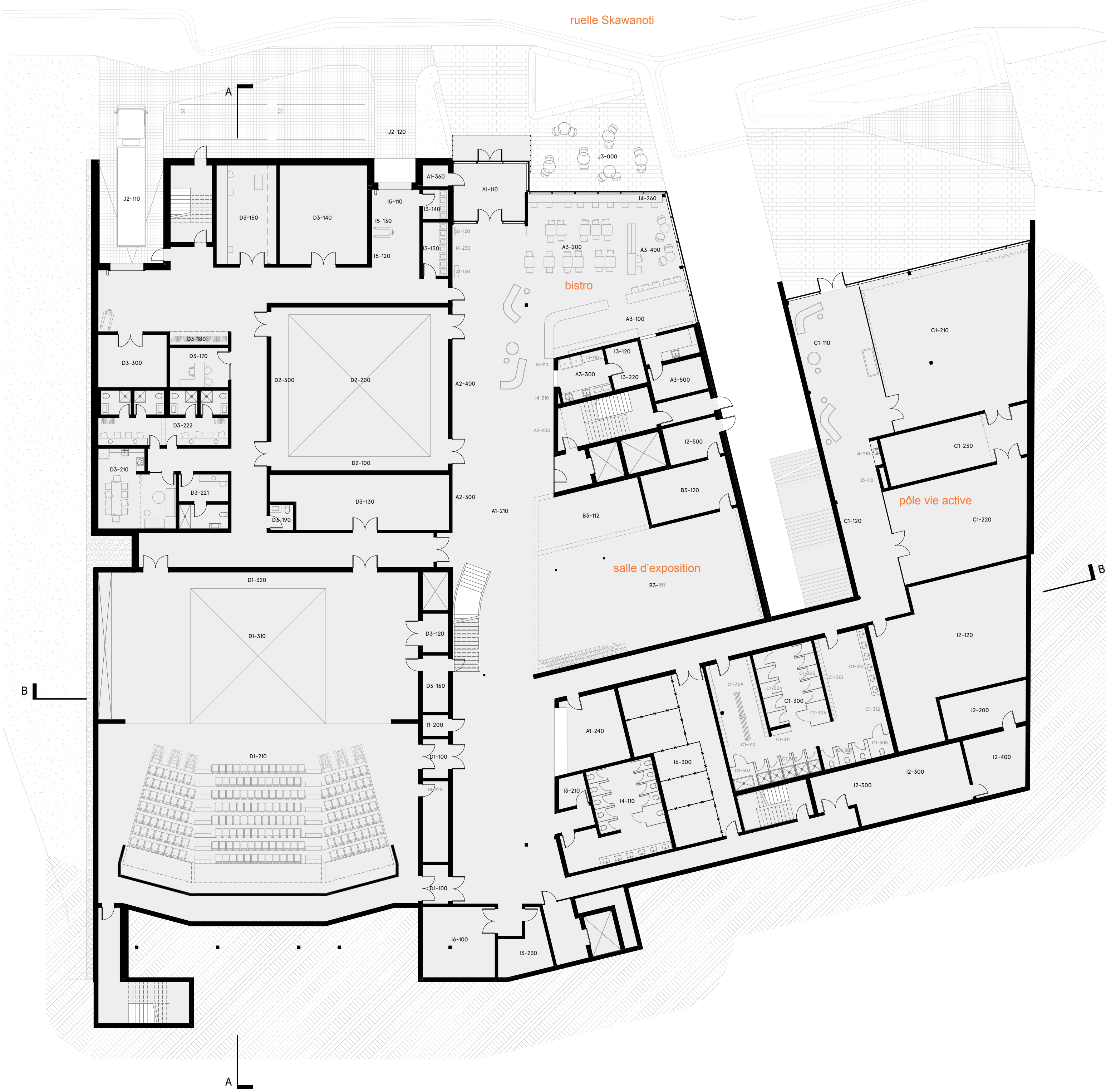
NIVEAU 00 rez-de-jardin ÉCHELLE 1 : 200
