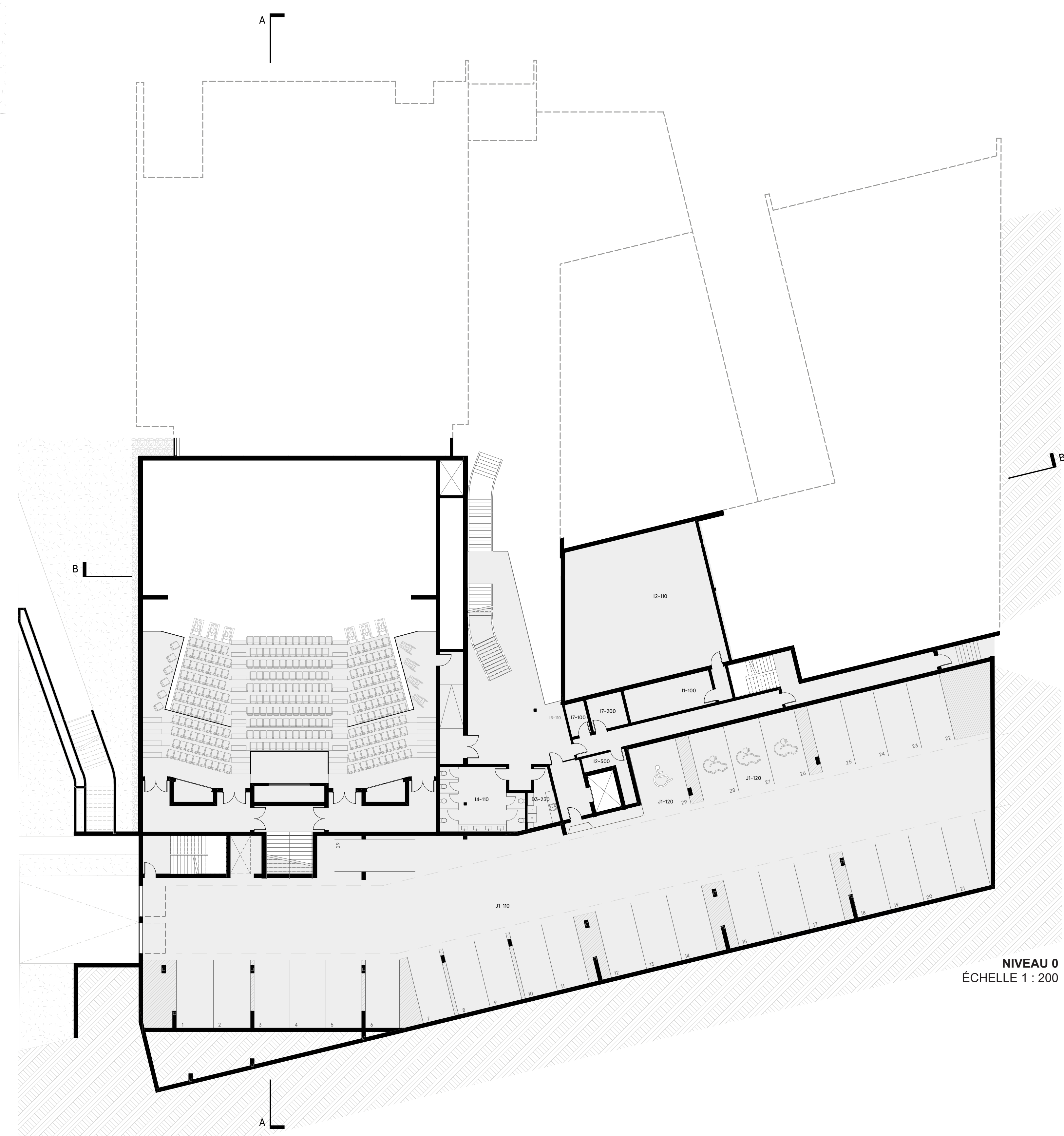
NIVEAU 00 rez-de-jardin ÉCHELLE 1 : 200
