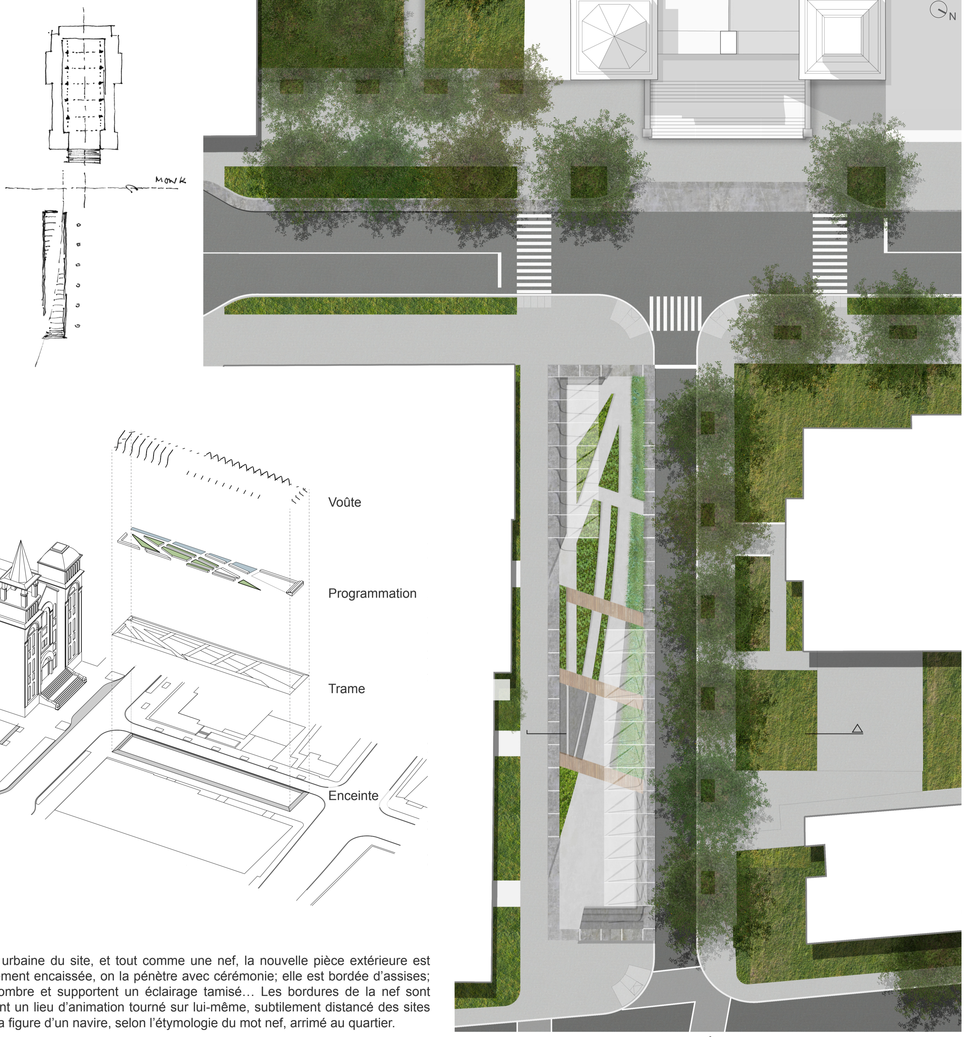
Vue en plan de la zone d'intervention - Échelle 1:200
