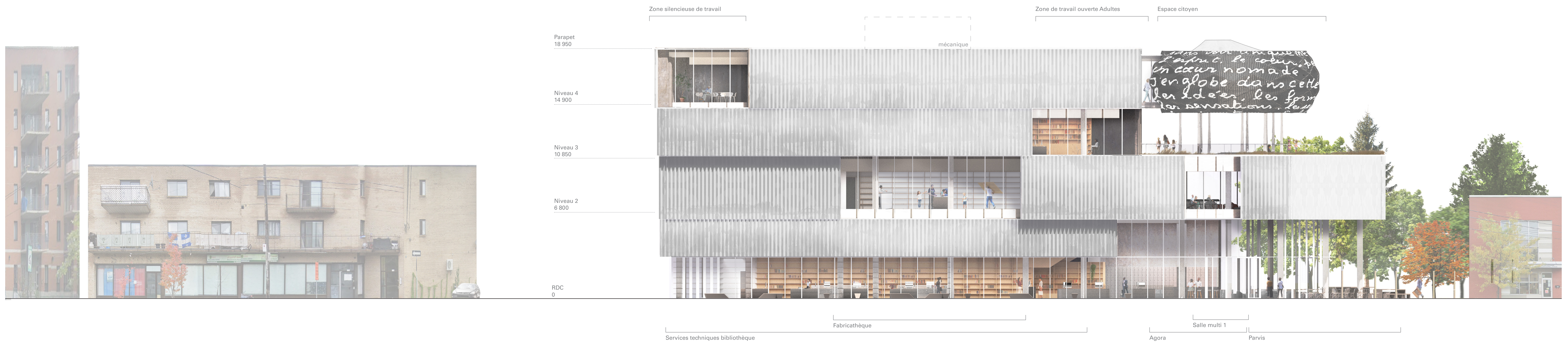
Elevation Boulevard Henri-Bourassa - Ouest 1:100
