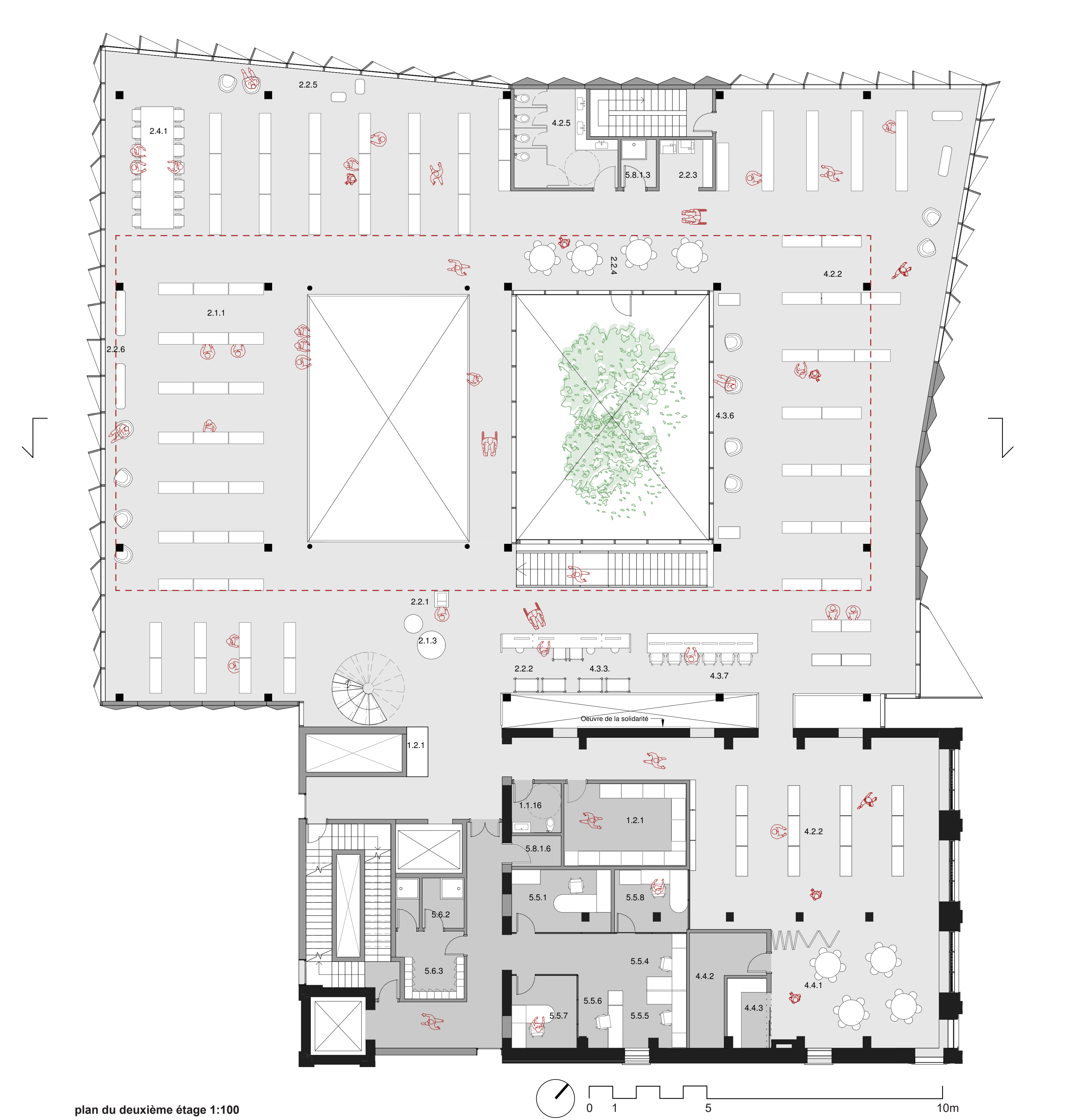
plan du deuxième étage 1:100
