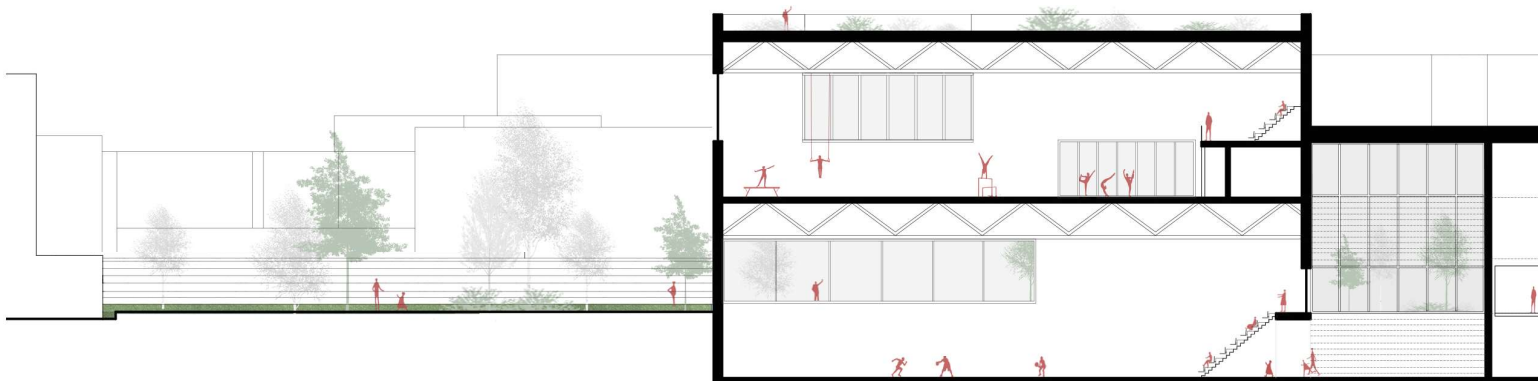
COUPE LONGITUDINALE (GYM+PALESTRE)
