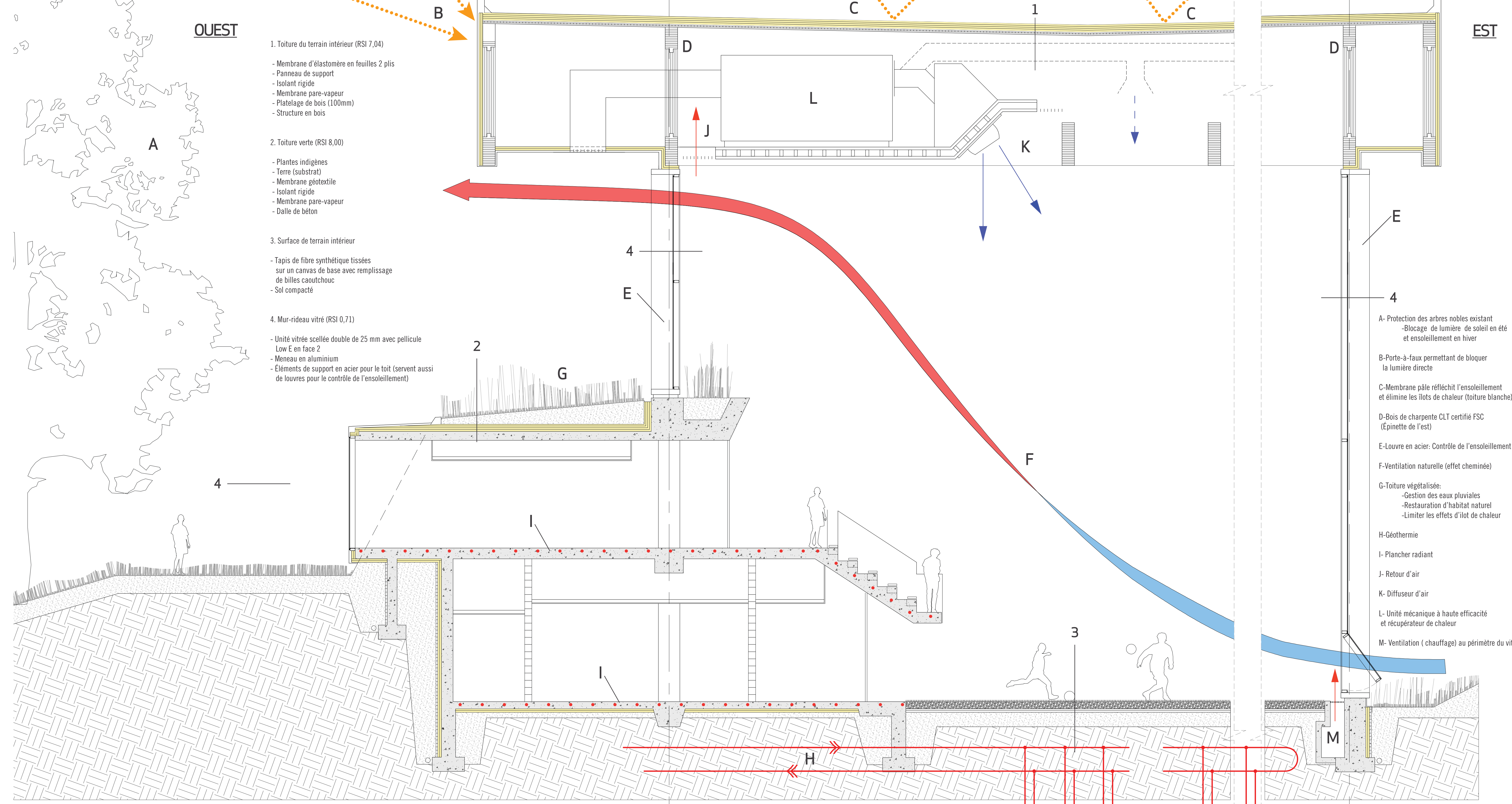
COUPE DÉTAILLÉE DE L'ENVELOPPE 1:50
