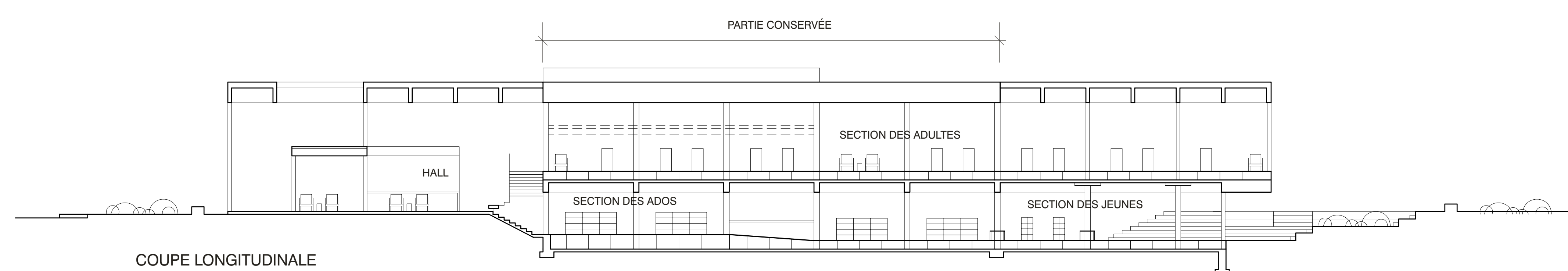
COUPE LONGITUDINALE 1:150
