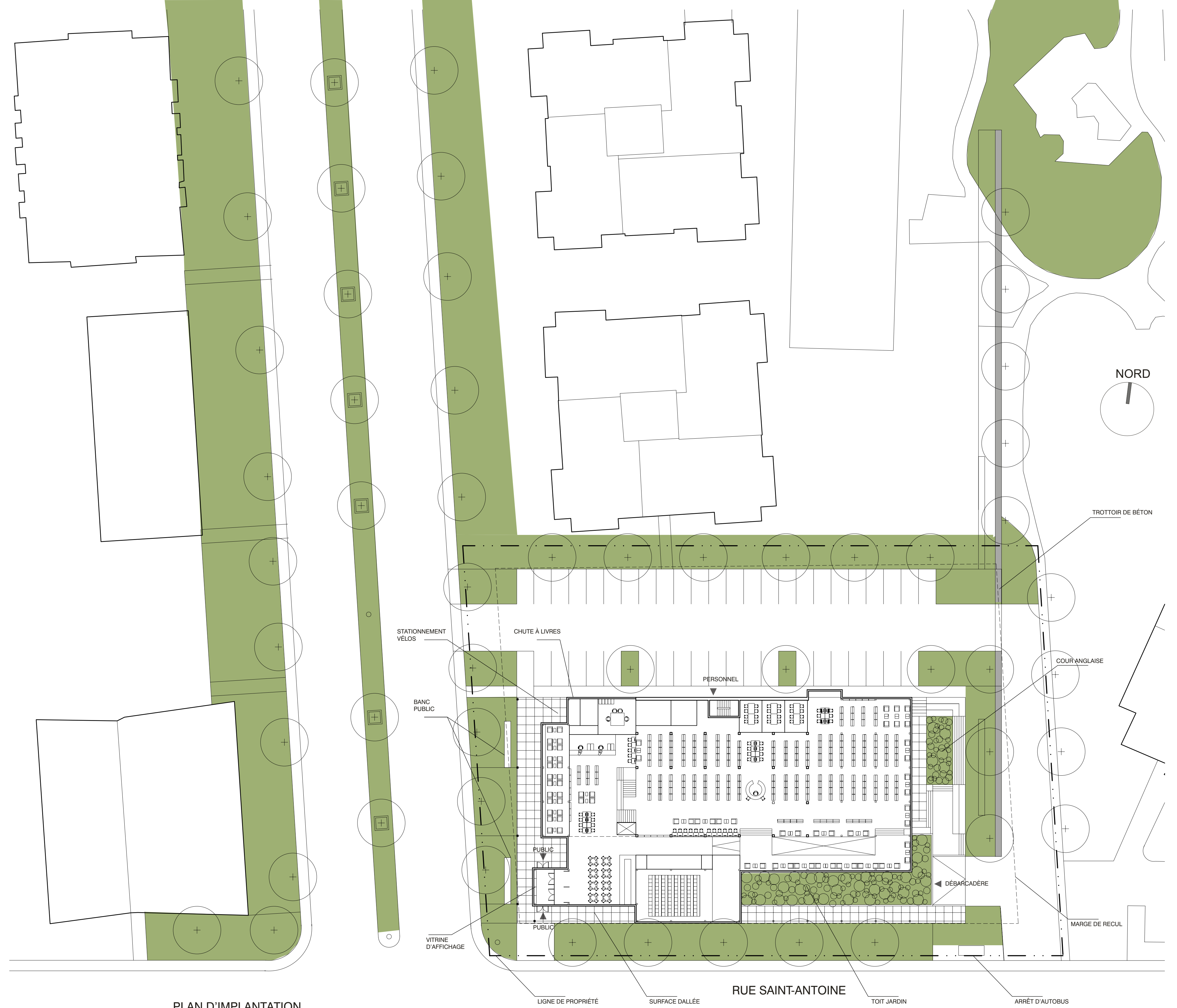
PLAN D'IMPLANTATION 1:300
