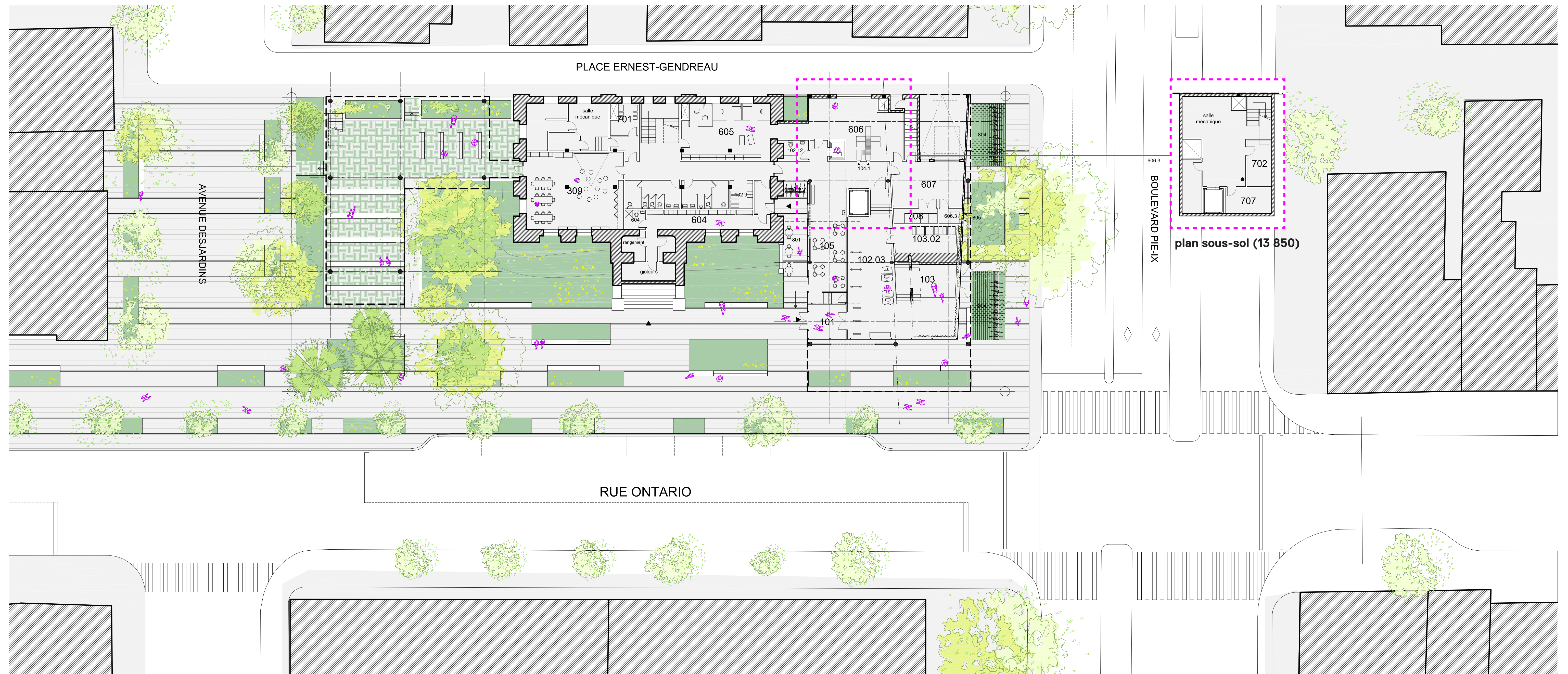
plan niveau rue (19 000) _ 1:200
