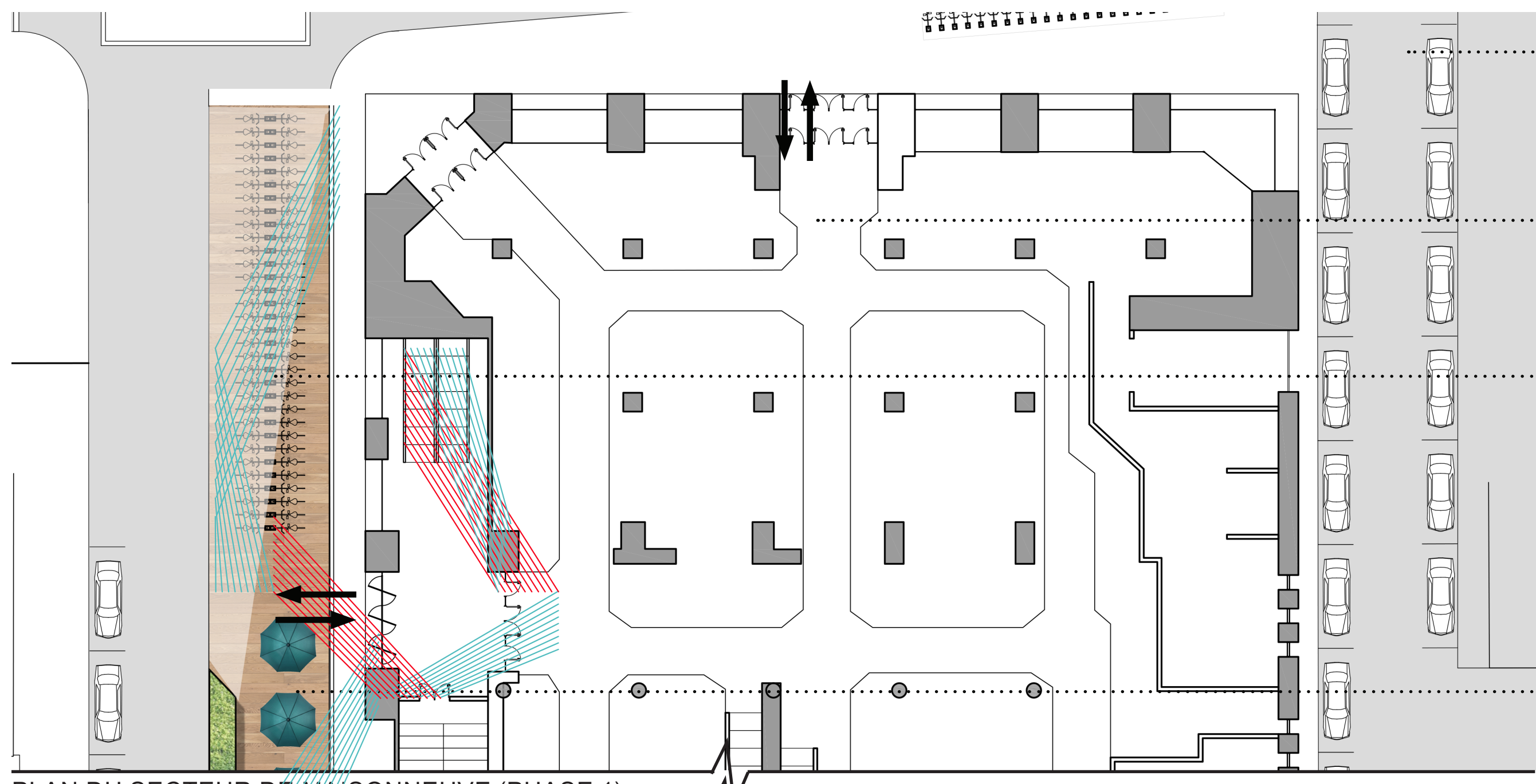
PLAN DU SECTEUR DE MAISONNEUVE (PHASE 1)
