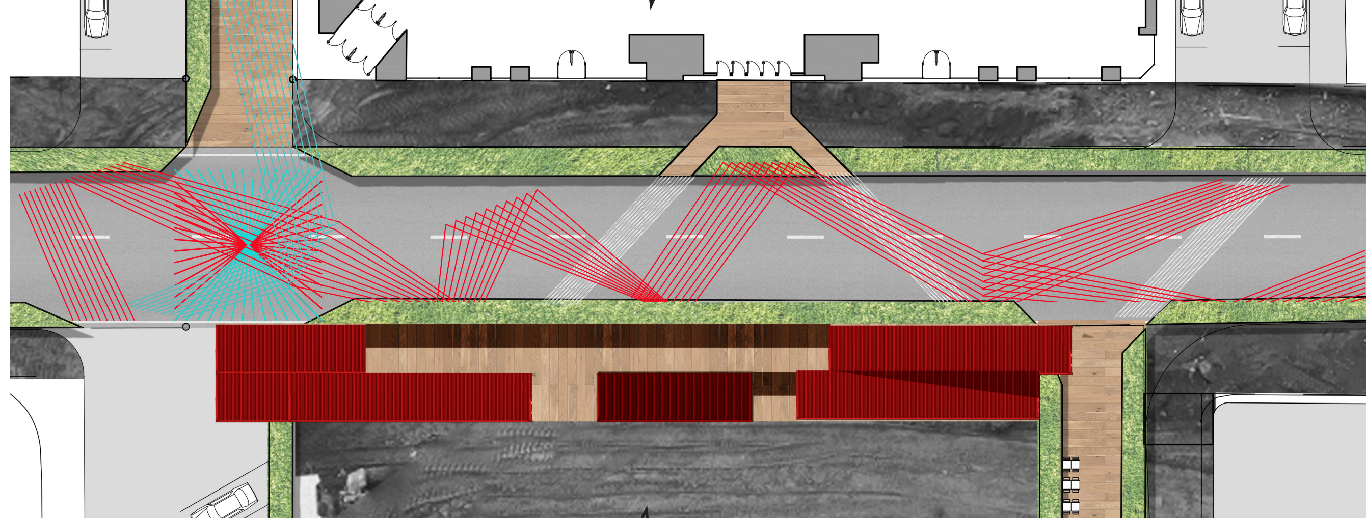
PLAN DU SECTEUR SQUARE PHILLIPS (PHASE 1)
