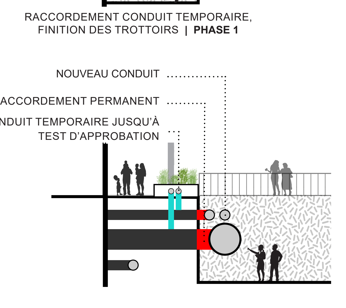
DÉPLACEMENT BAC - CONDUIT SUR SURFACE FINIE | PHASE 1
