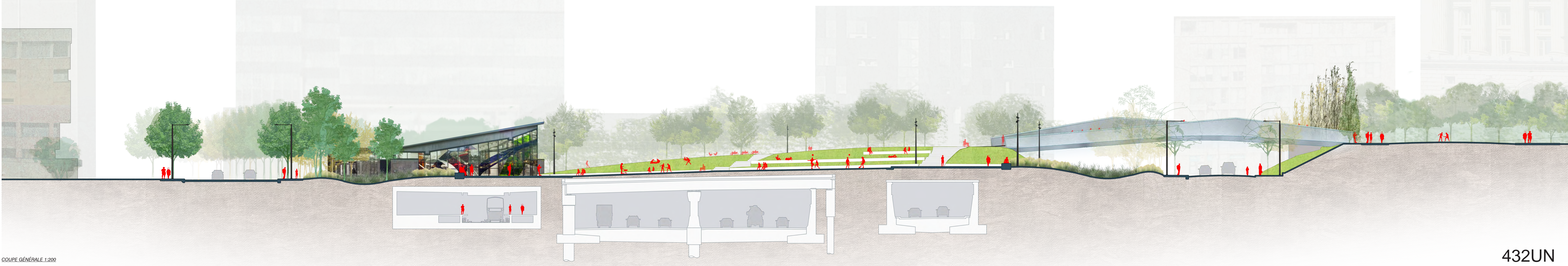
COUPE GÉNÉRALE 1:200
