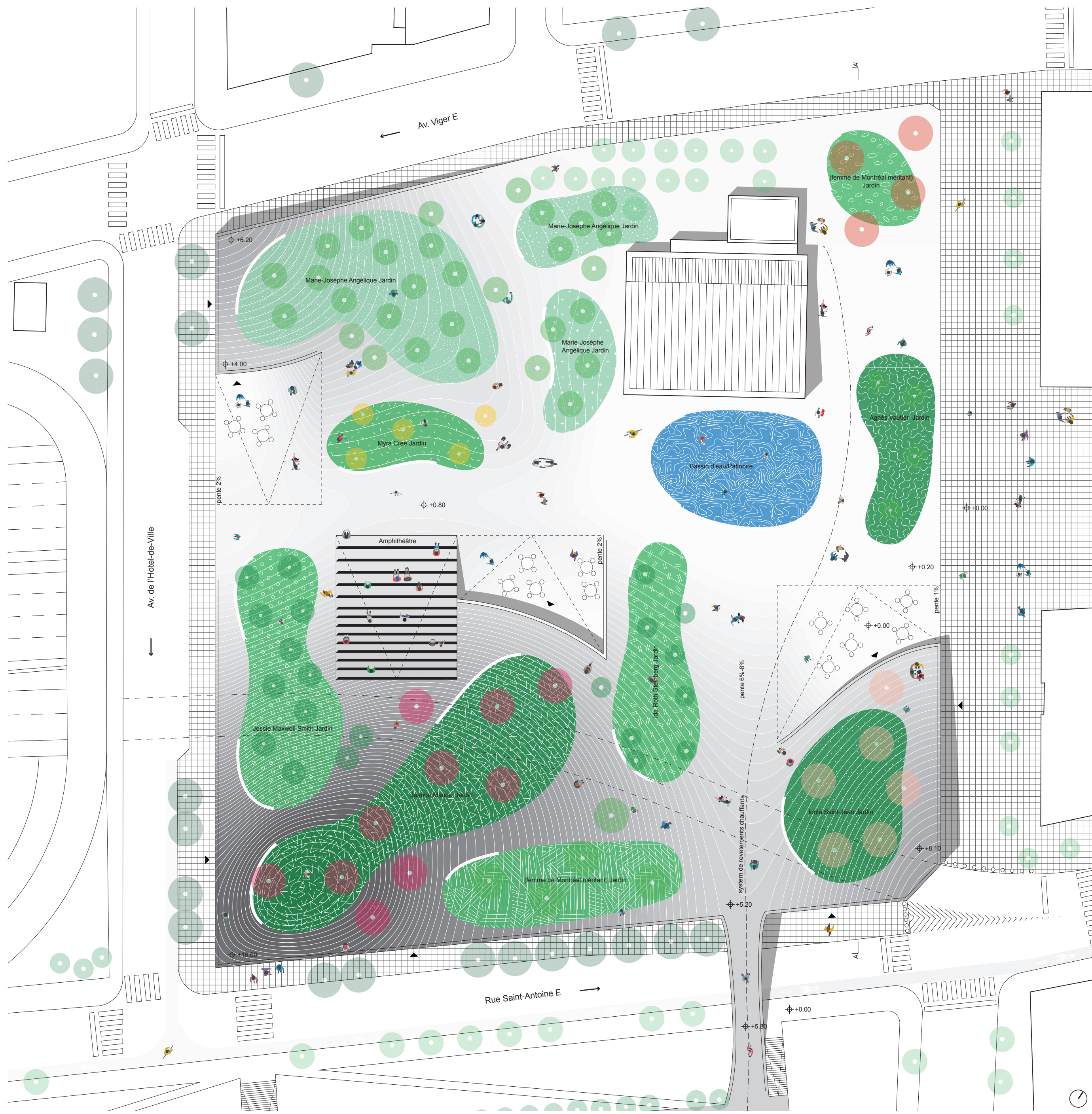
Plan masse 1:500
