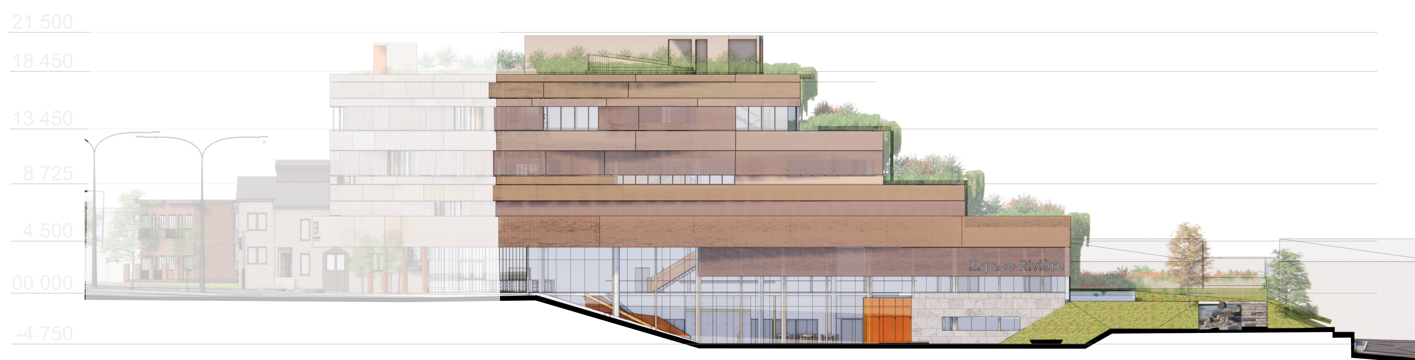
ÉLÉVATION NORD-EST
