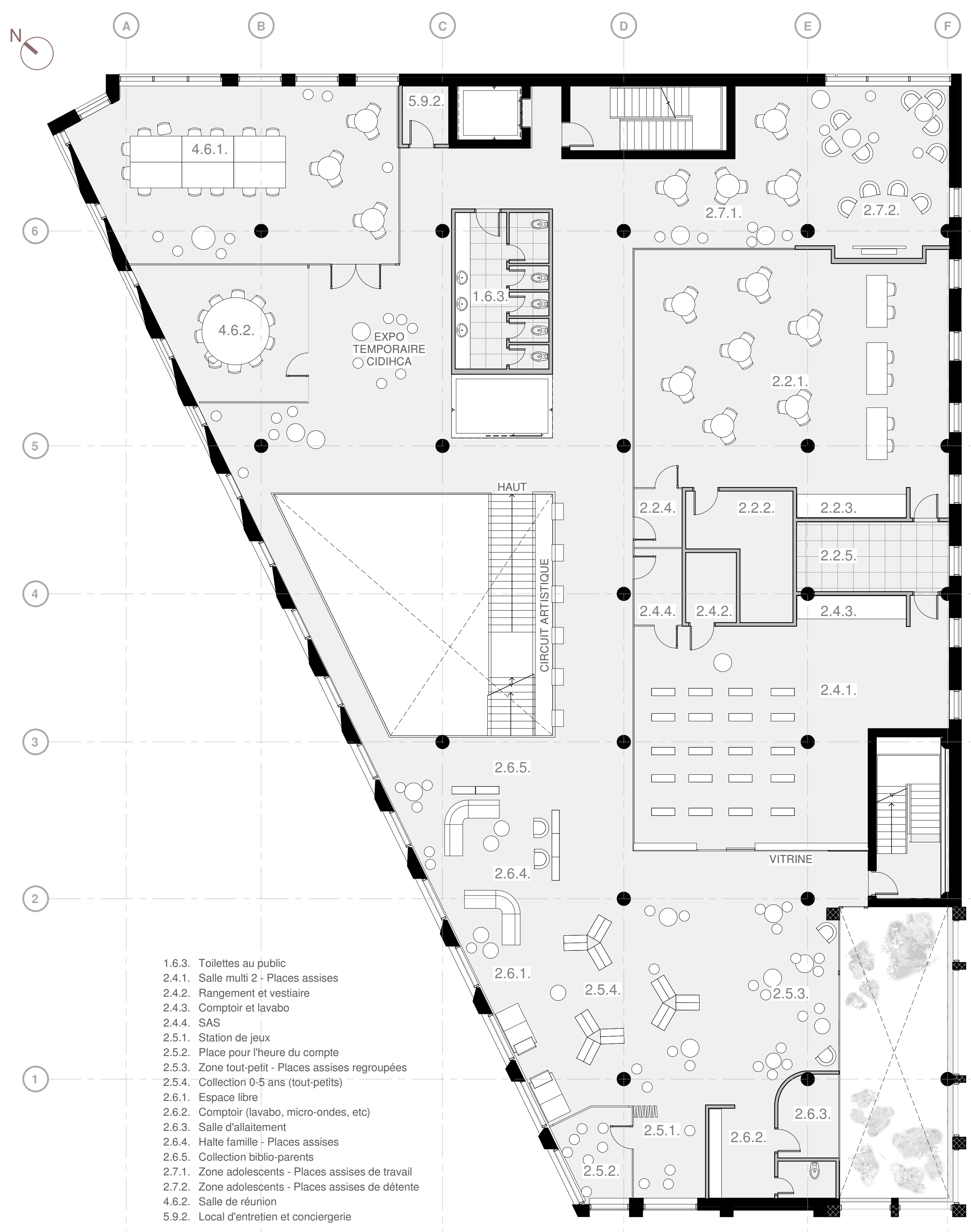
NIVEAU 1 | 1:100
