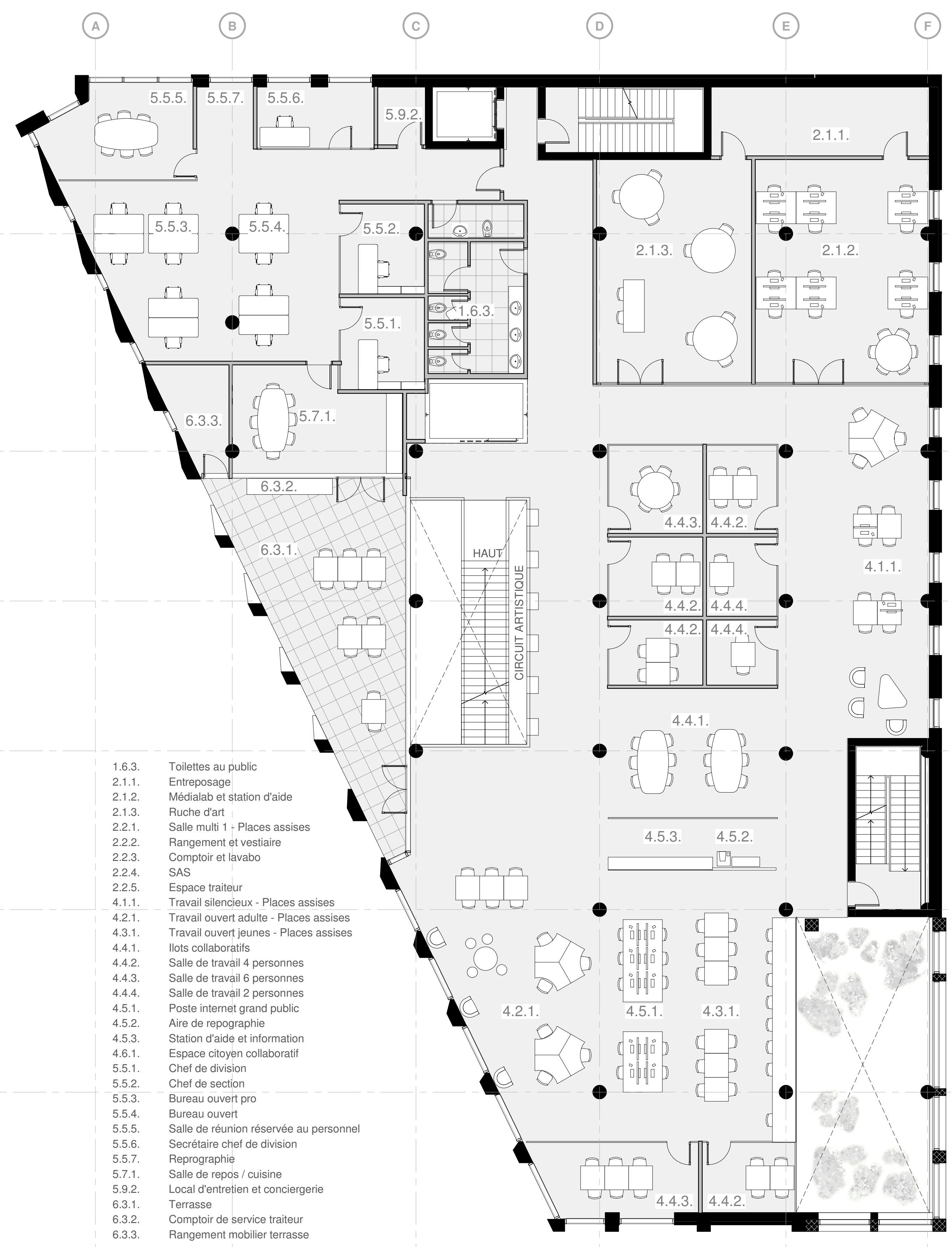
NIVEAU 2 | 1:100
