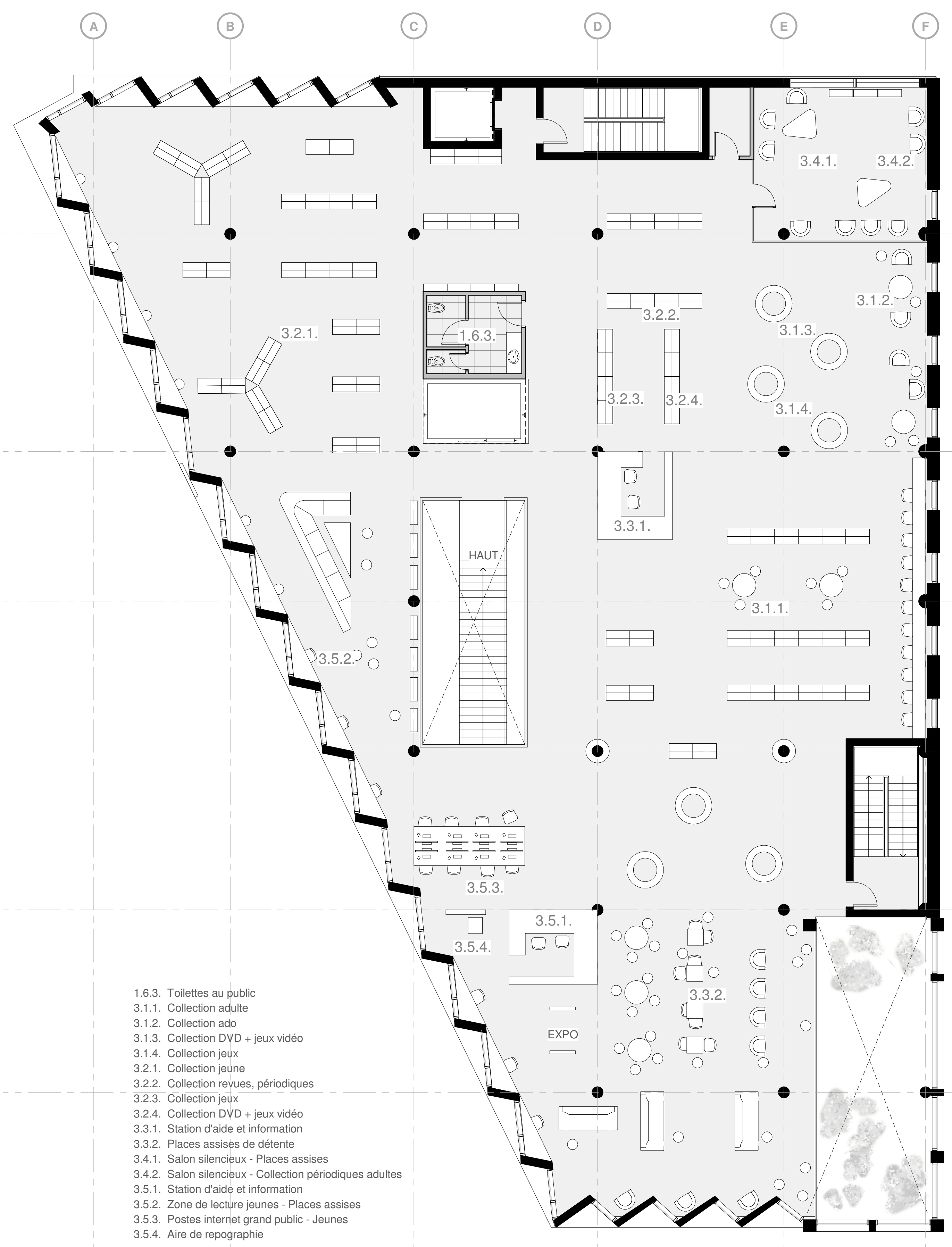
NIVEAU 3 | 1:100
