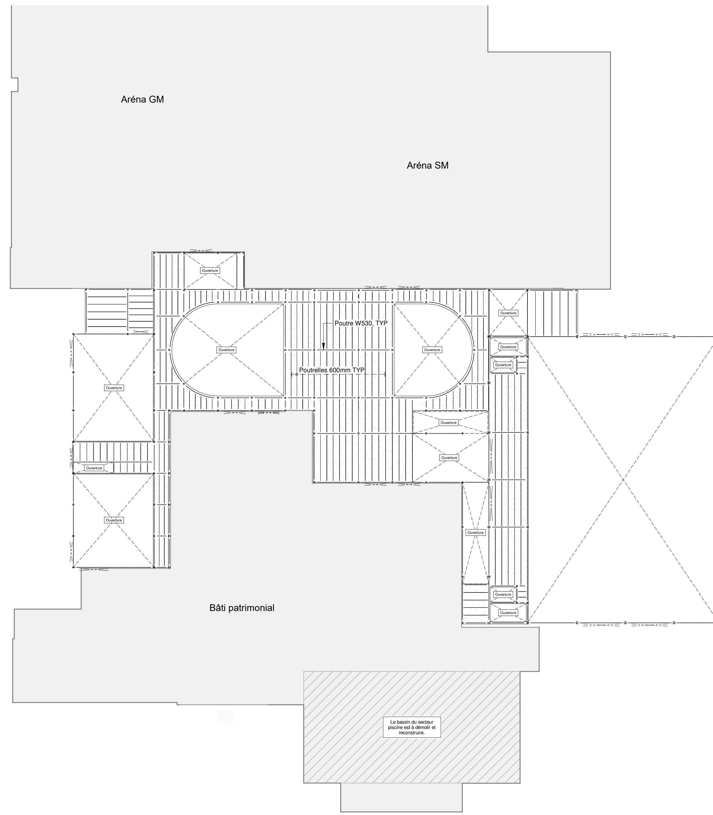
Plan de structure - Rez-de-jardin échelle : 1 : 400
