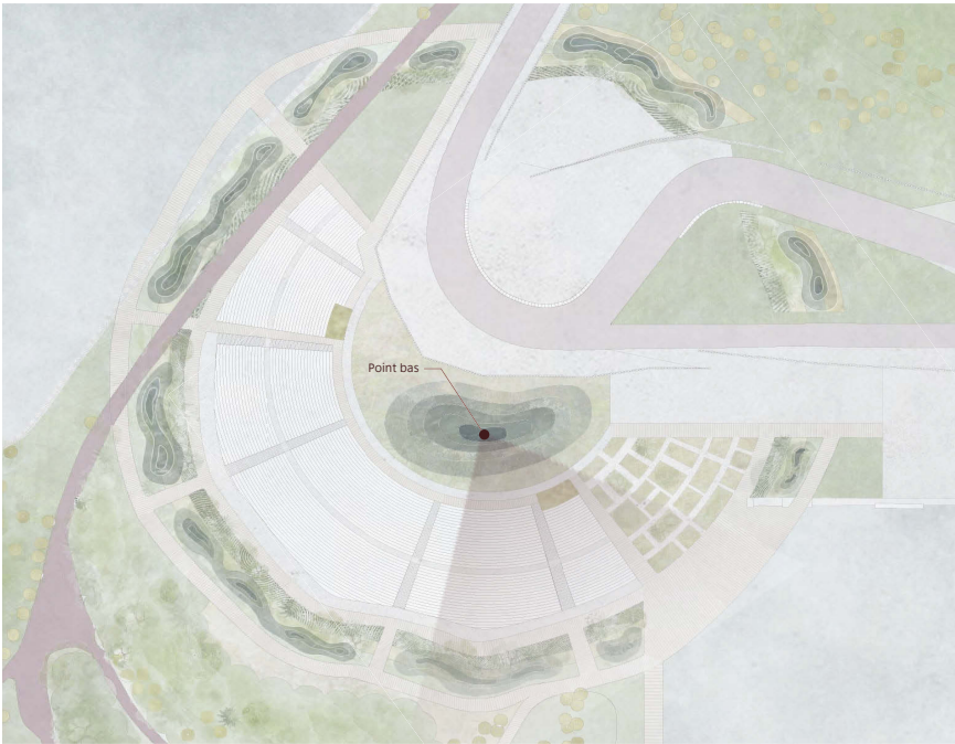
Plan du secteur des courbes Senna - Biorétention
