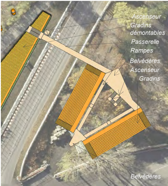
Plan schématique de la tour de gradins à l'intérieur de la courbe principale, secteur Sud
