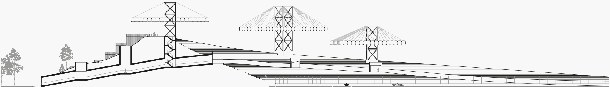
Coupe schématique des gradins — Galeries, circulation verticale et tours plateformes
