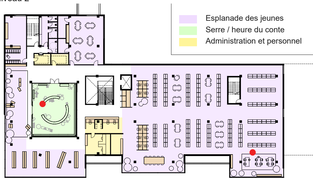
plan niveau 1
