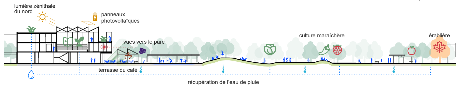
Coupe schématique de la bibliothèque et du parc
