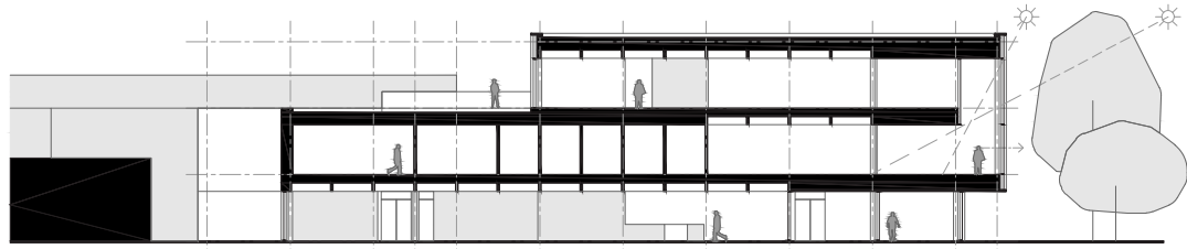
Coupe transversale C-C
